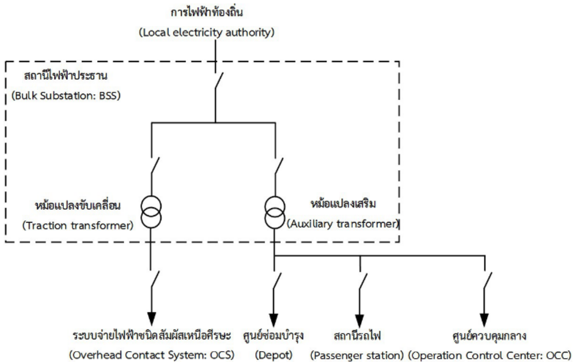
รูปที่ 2 ตัวอย่าง single line diagram สำหรับการออกแบบระบบการจ่ายไฟฟ้ากระแสสลับ
