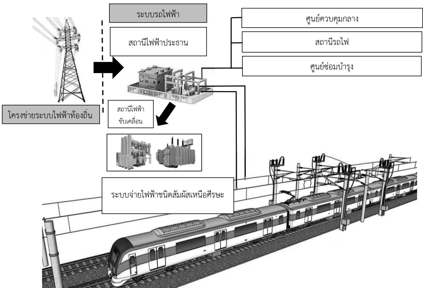
รูปที่ 1 ภาพรวมของระบบจ่ายไฟฟ้ากระแสสลับสำหรับรถไฟสายประธาน
